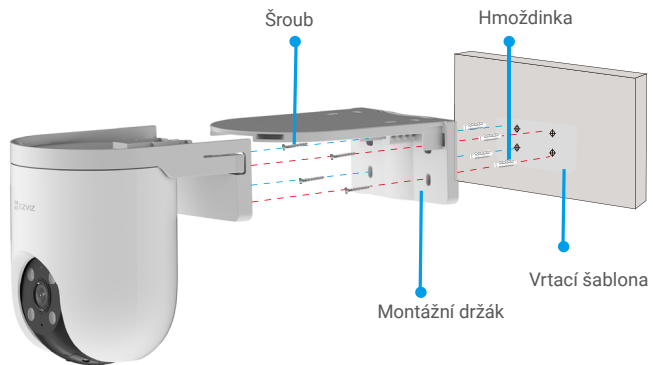
Obr. 2 Montáž na zeď
