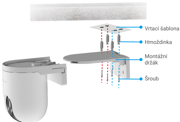
Obr. 1 Montáž na strop
